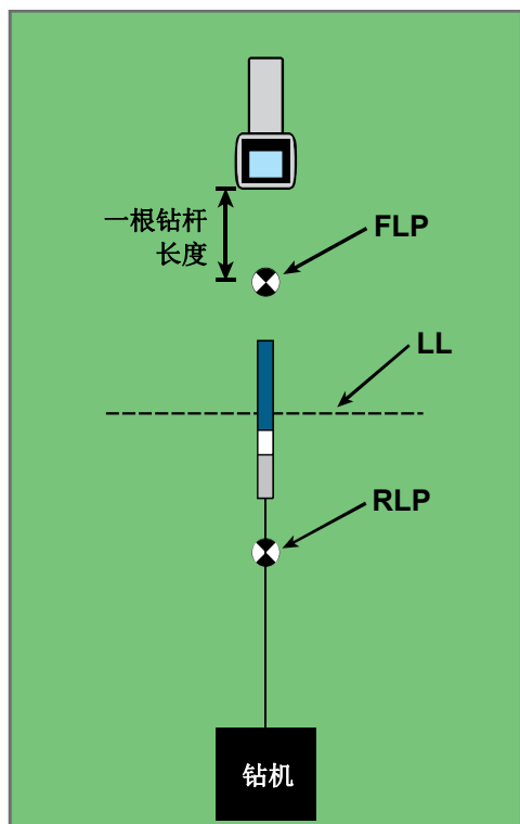
直线钻进情形下的“飞行”跟踪
