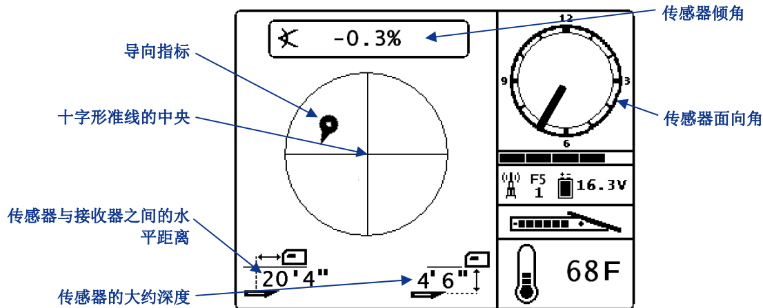
远程显示器屏幕上示出的目标指引
