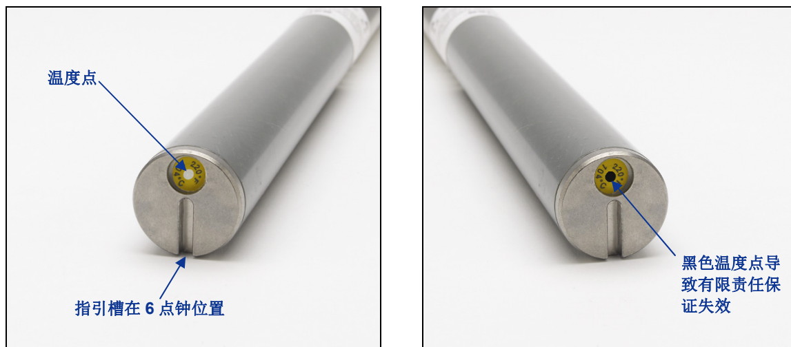
显示出温度点的传感器前端盖、指引槽以及黑色温度点
