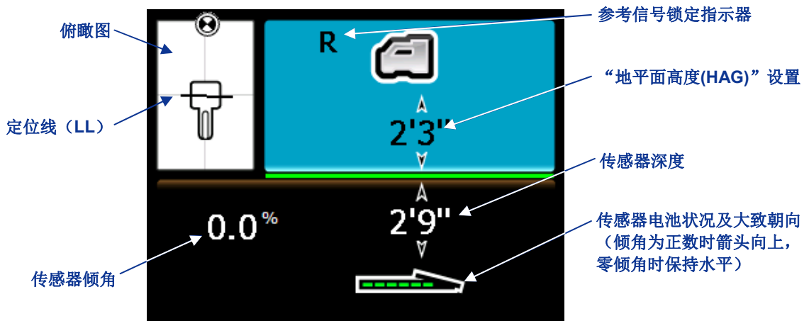
HAG 启用、接收器位于定位线上情形下的接收器深度模式屏幕（扣住点击开关）
