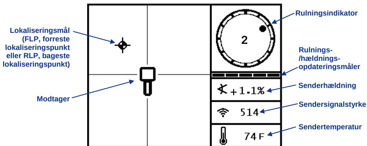
Modtagerens lokaliseringstilstandsskærm med sender inden for rækkevidde (trigger ude)
