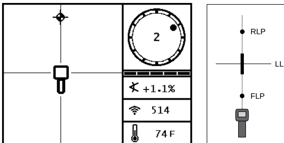
Modtagerens skærm sporer "i farten"
