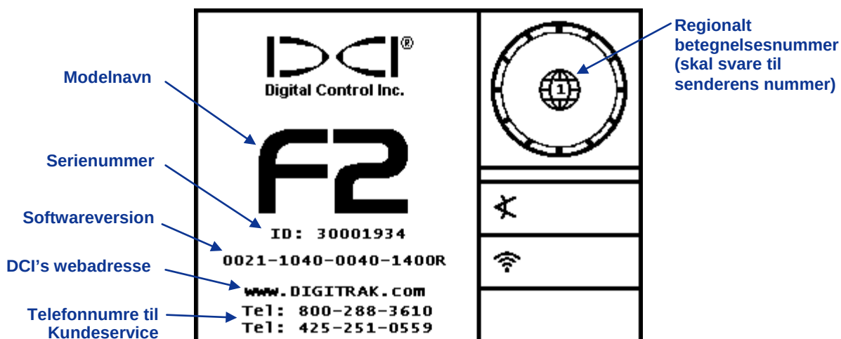
Modtagerens startskærm
