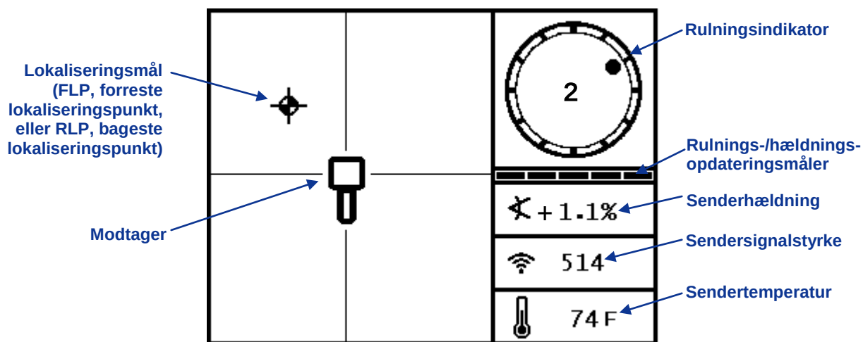
Modtagerens lokaliseringstilstandsskærm
