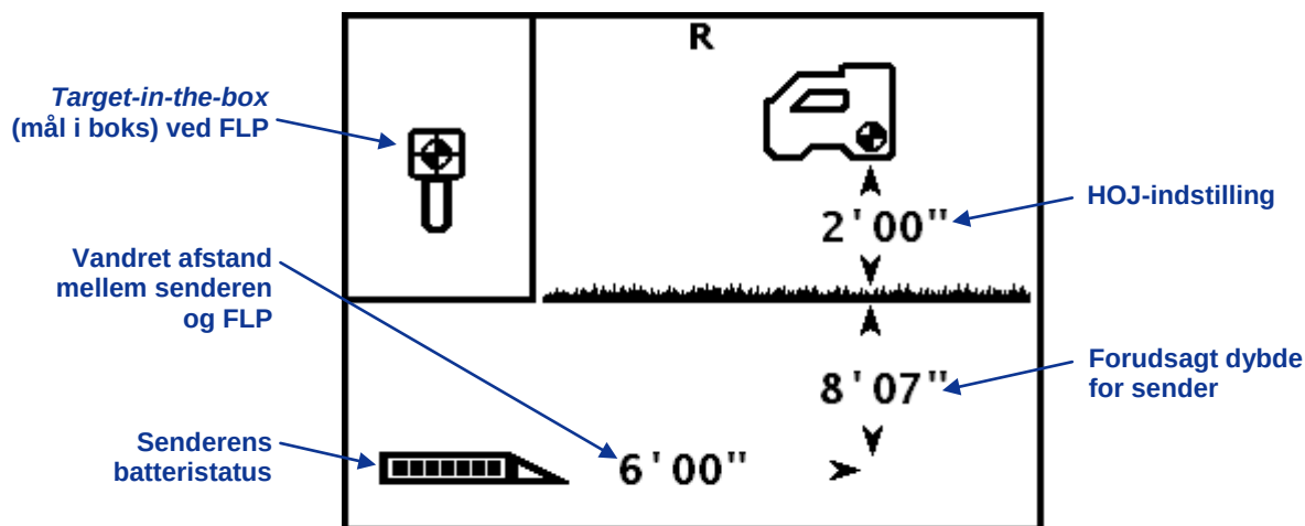
Modtagerens skærm til forudsagt dybde ved FLP med HOJ aktiveret (trigger inde)
