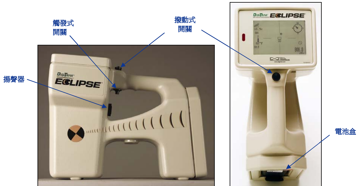
Eclipse 接收器的側面圖（左邊）和俯視圖（右邊）
