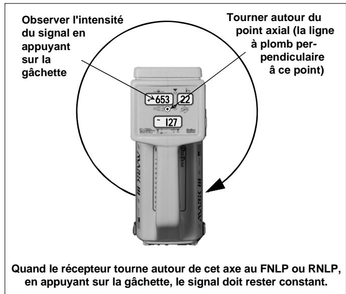
Méthode de confirmation de la position
