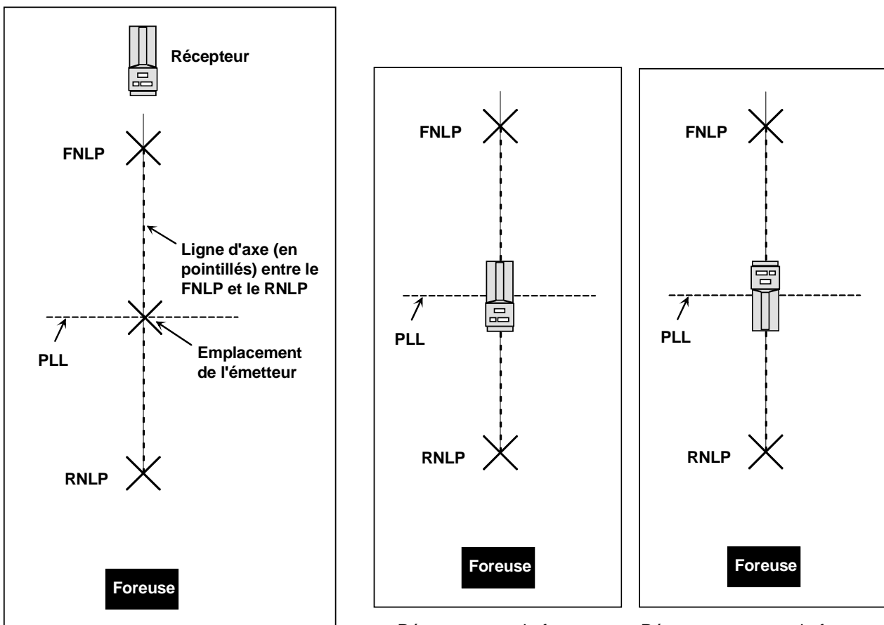
Détermination de l'emplacement de l'émetteur
