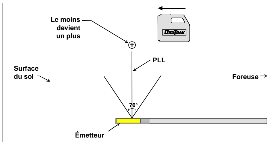
Détermination de la ligne de repère positive (PLL) à partir de la foreuse
