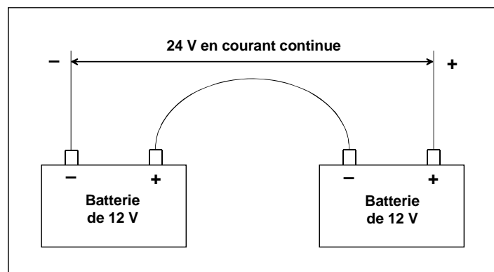
Branchement des batteries en série
