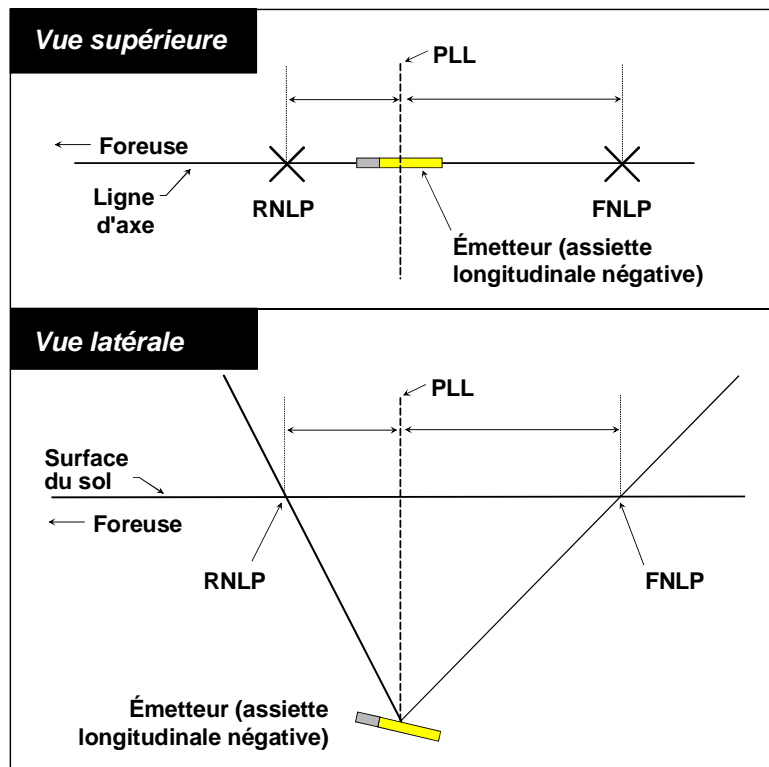
Effet de l'assiette longitudinale sur la distance entre le FNLP, le RNLP et la PLL - Il faut noter que le RNLP et le FNLP sont à des distances différentes de la PLL quand l'émetteur a une assiette longitudinale négative (comparer au schéma de la page précédente où l'émetteur est horizontal).
