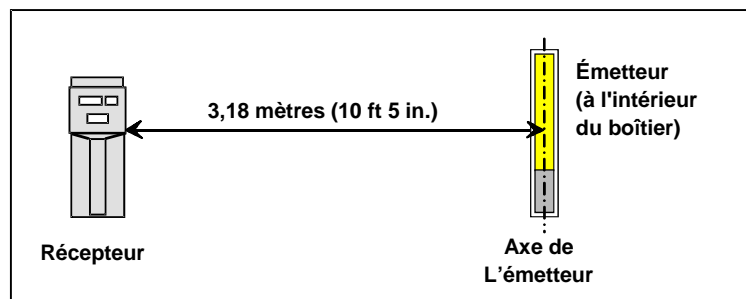
Étalonnage sur un point
