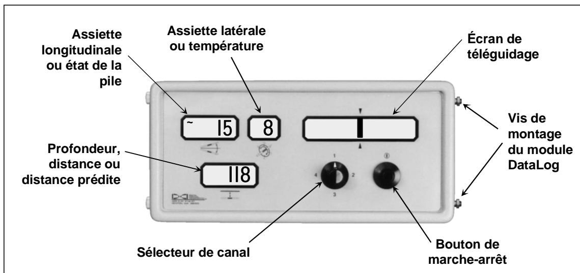
Appareil de télaffichage
