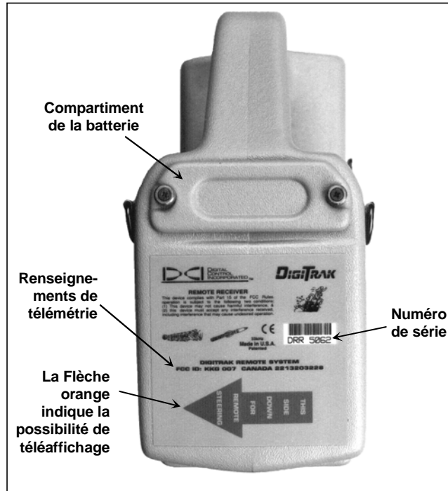
Récepteur DigiTrak– Arrière montrant les renseignements d'identification
