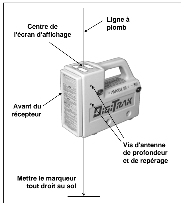
Ligne à plomb de l'antenne
