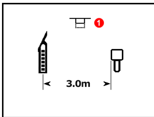
Kalibreringsprompt
