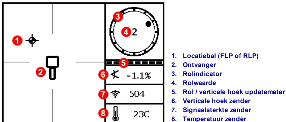
Lokalisatiescherm met zender binnen bereik
