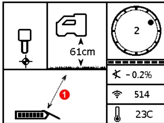
Het diepteschermb van de ontvanger met HAG ingeschakeld (niet op FLP, RLP of LL)
