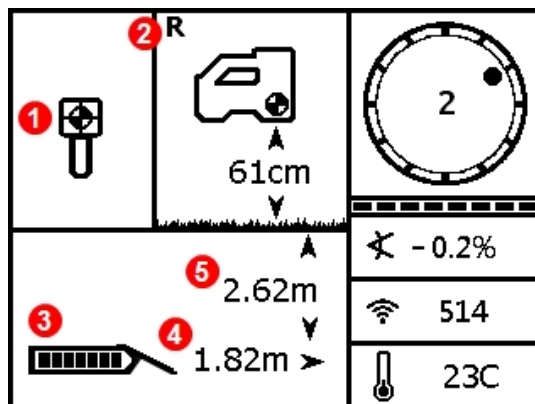
Schermb Voorspelde diepte op FLP met HAG ingeschakeld
