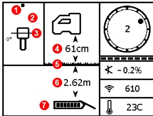
Diepteschermb op LL met HAG ingeschakeld
