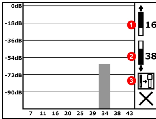
Grafiek van frequentie-optimalisator tijdens het scannen
