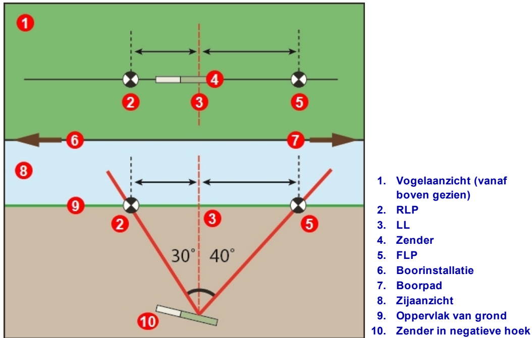
Effect van negatieve hoek op afstand tussen FLP, RLP en LL
