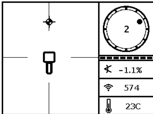
Scherm van ontvanger “On-the-Fly” lokaliseren
