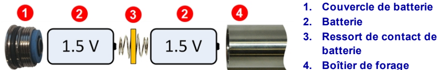
Installation de batteries type C avec ressort de contact de batterie
