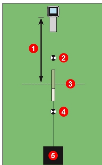
A vevő elhelyezése a célzott irányításhoz
