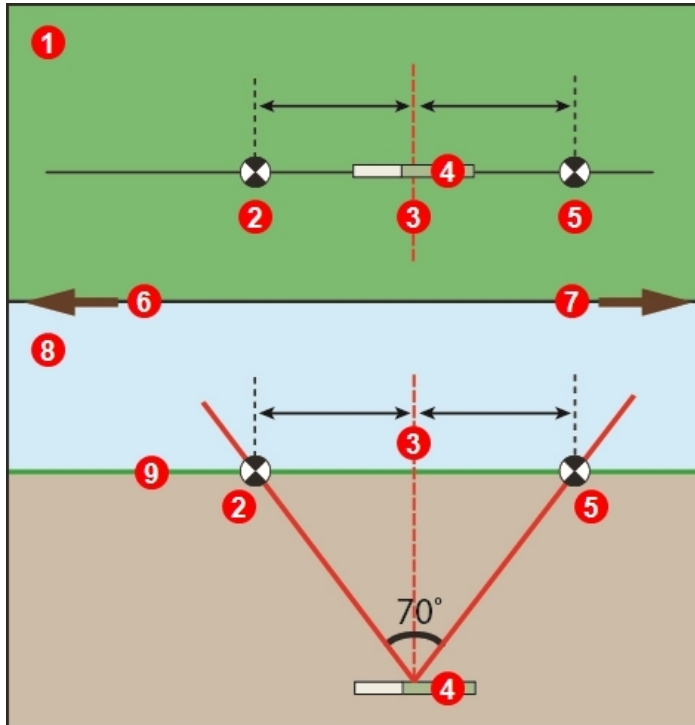
Az FLP, RLP és LL geometriája felül- és oldalnézetből
